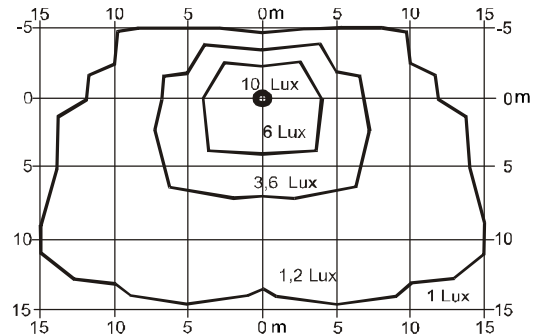
Característica luminosa desde un punto luminoso de 4m de altura
